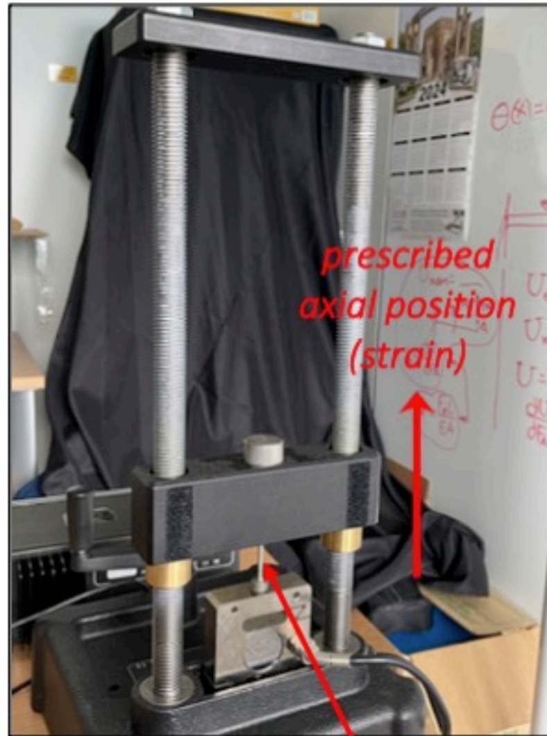
Test rig
